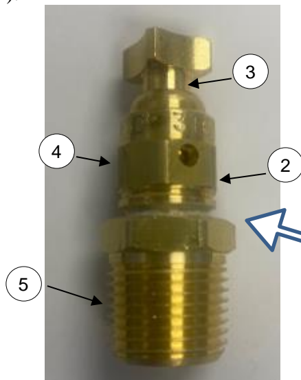
Typical Bleeder valve to replace removable drain plug on a typical meter | Vanne de purge typique pour remplacer le bouchon de vidange amovible sur un compteur typique
