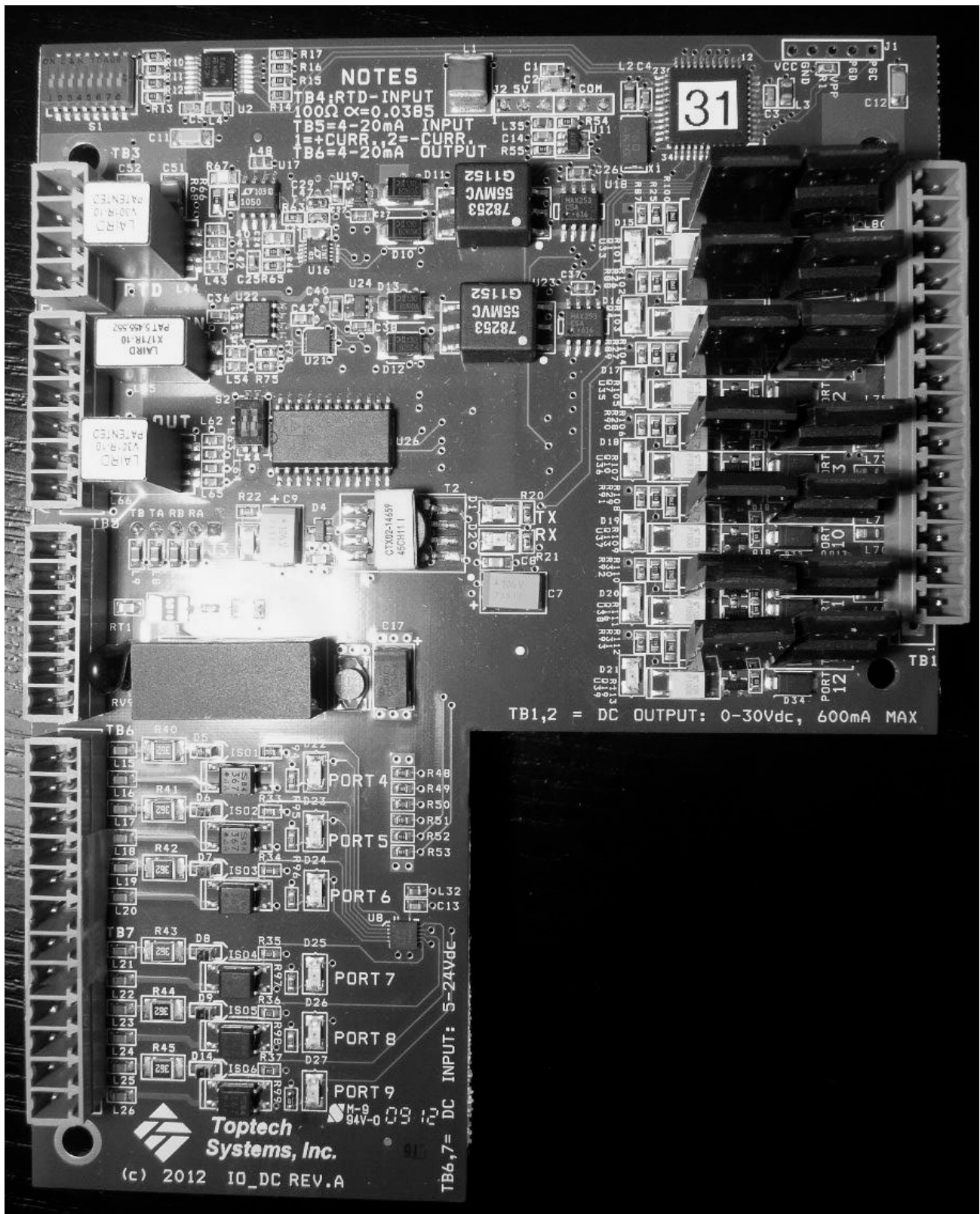
Fig. 15 : Single Meter I/O Board (DC MOSFETs) / carte entrée/sortie pour un compteur (Transistor MOS c. c.)
