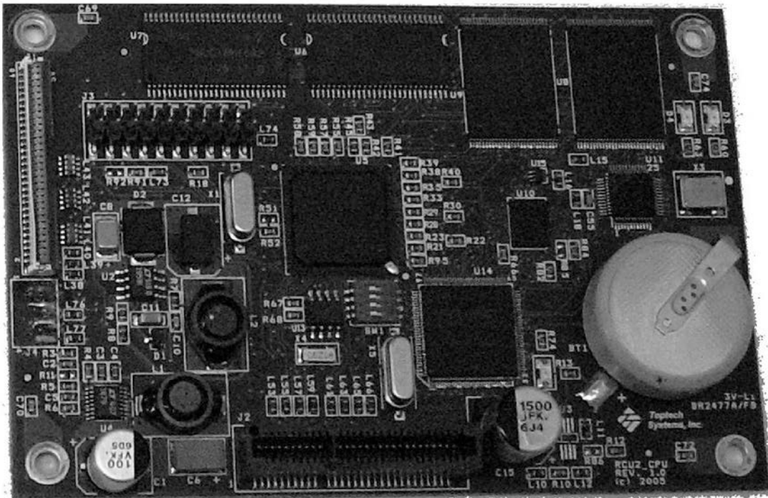
Fig. 10 : Old CPU card / Ancienne carte UC
