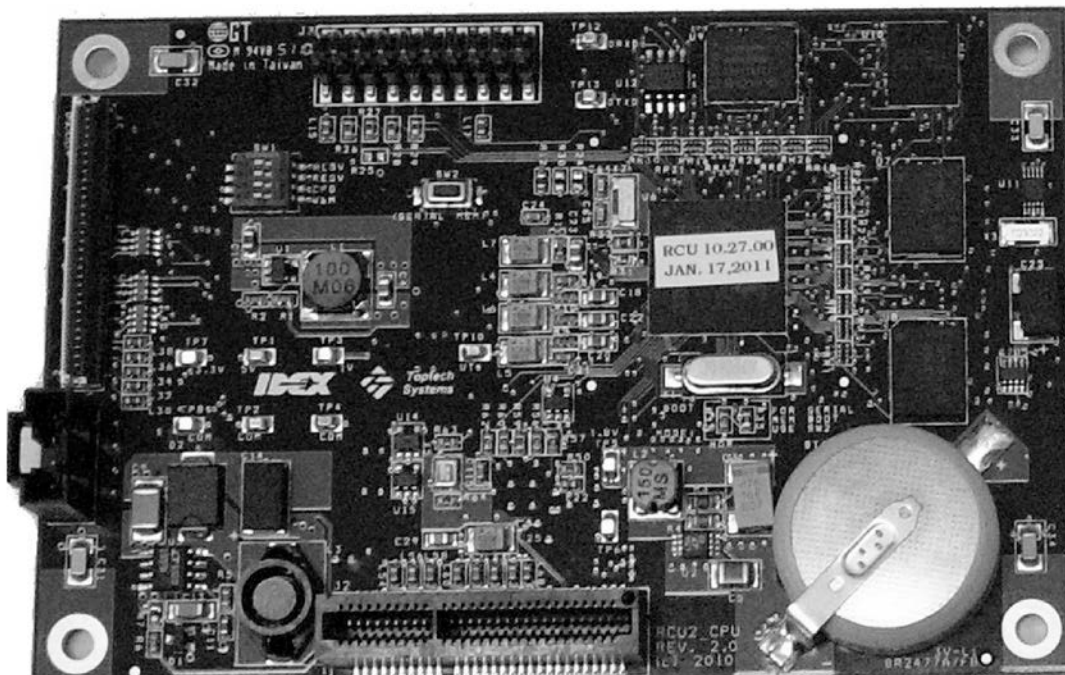
Fig. 11 : New CPU Card / Nouvelle carte UC
