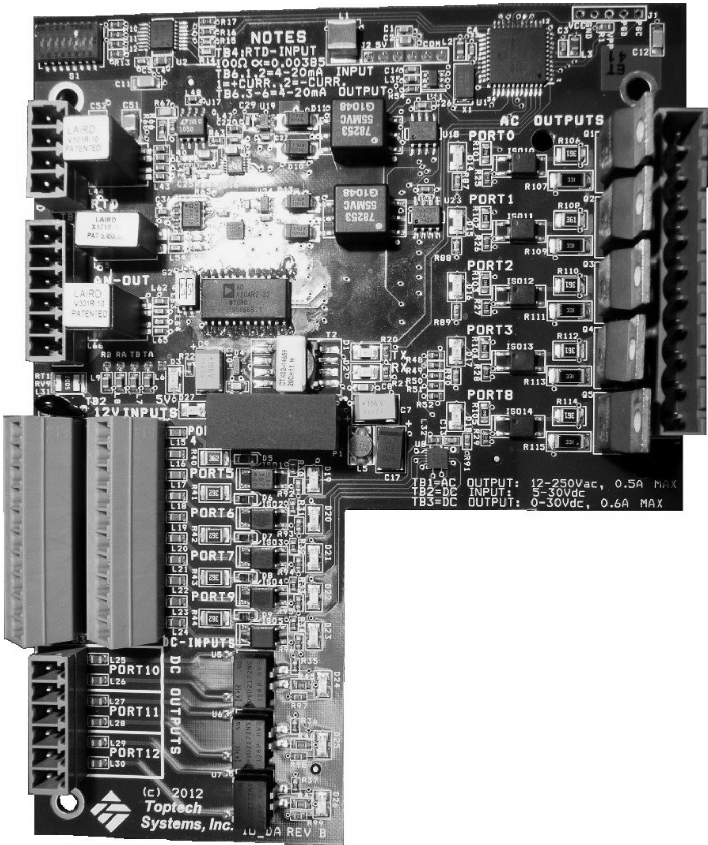
Fig. 14 : Single Meter I/O Board (AC Triacs) / carte entrée/sortie pour un compteur (Triacs c. a.)
