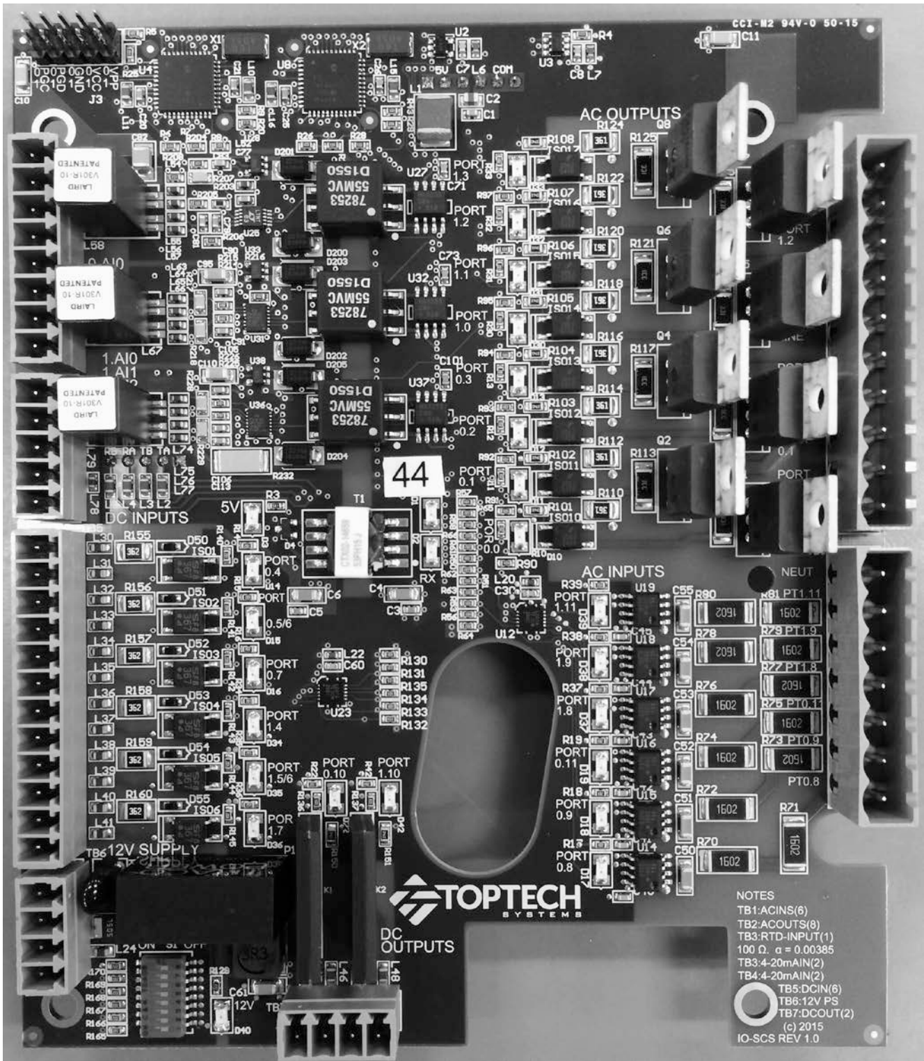
Fig. 16: SCS I/O board with multiplexer /SCS carte entrée avec multiplexeur
