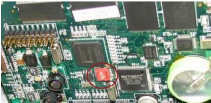
Figure 9 DIP switches for Program / W&M access; rev. 1.0 on old CPU board (left) and rev. 2.1 on new CPU board (right) | Interrupteurs DIP pour l'accès du mode « Program » et « W&M »; rév. 1.0 sur l'ancienne carte de CPU (gauche) et rév. 2.1 sur la nouvelle carte CPU (droit)
