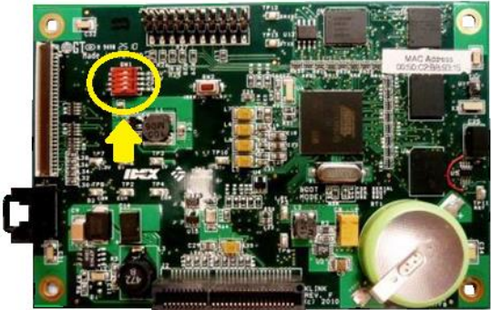
Figure 9 DIP switches for Program / W&M access; rev. 1.0 on old CPU board (left) and rev. 2.1 on new CPU board (right) | Interrupteurs DIP pour l'accès du mode « Program » et « W&M »; rév. 1.0 sur l'ancienne carte de CPU (gauche) et rév. 2.1 sur la nouvelle carte CPU (droit)
