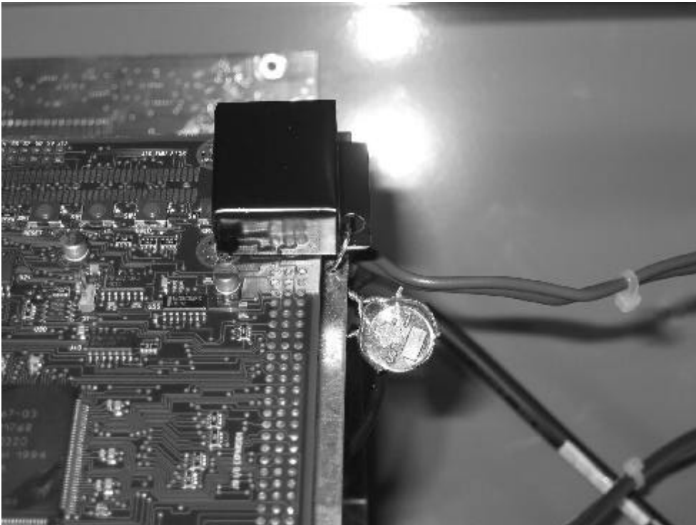
Fig. 3: Switch Cover Seal of the iGEM register circuit board / Sceau du couverture de l'interrupteur de la carte de circuits imprimés du totalisateur iGEM
