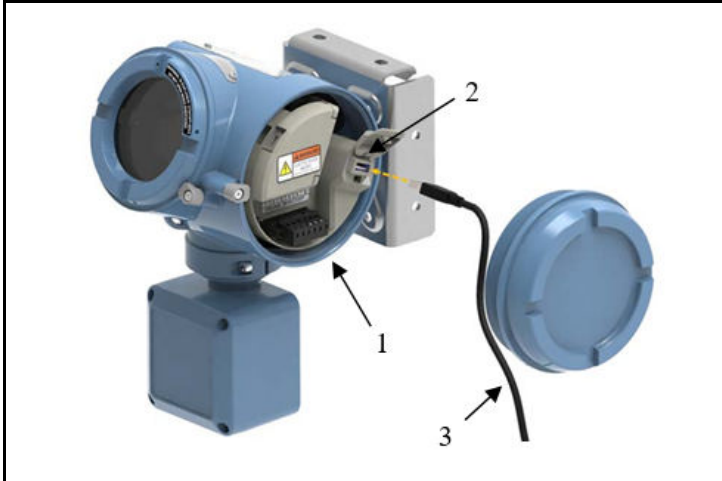
Figure 14: Accessing 4700 parameters using ProLink: | Accès aux paramètres de 4700 en utilisant le logiciel ProLink :
