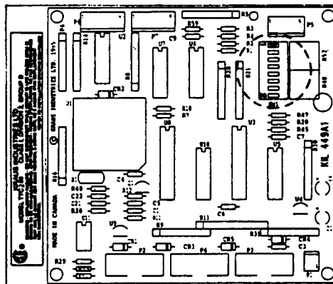
SW1 - eight DIP switches / huit commutateurs DIP
