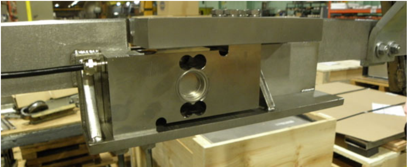
Load cell mounting / Montage de la cellule de pesage
