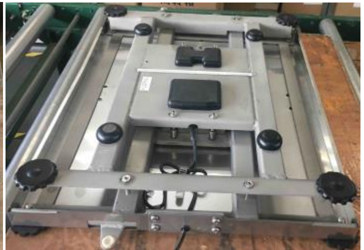
Typical Sub-platter Models S-UK or S-UKS / Sous-plateau typique modèles S-UK ou S-UKS
