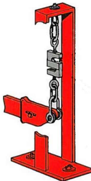
Typical load cell mount / Montage de la cellule de pesage typique
