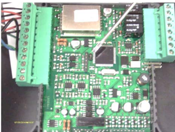
Calibration jumper position / Position du cavalier d'étalonnage
