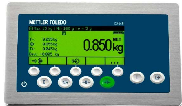
Typical Model ICS449-1 / Modèle typique ICS449-1
