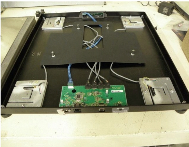
Typical sub-platter / Sous-plateau typique
