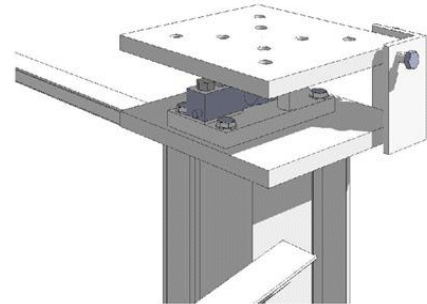
Typical stop for model LTBT-5000 / Butée typique pour le modèle LTBT-5000
