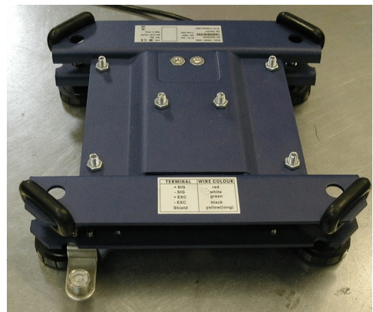
Typical model PBA220 sub-platter (stamped steel frame) / Sous plateau typique du modèle PBA220 (châssis en acier estampé)
