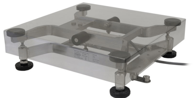
Typical model PBA226 sub-platter (10 kg, 25 kg, 50 kg and 100 kg capacities) / Sous-plateau typique du modèle PBA226 (capacités de 10 kg, 25 kg, 50 kg et 100 kg)
