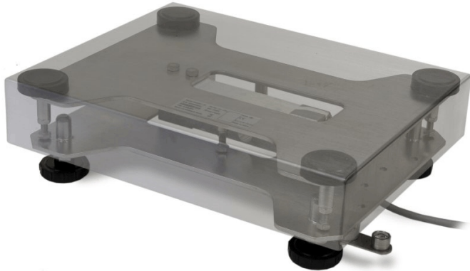
Typical model PBA226 sub-platter (2.5 kg and 5 kg capacities) / Sous-plateau typique du modèle PBA226 (capacités de 2.5 kg et 5 kg)
