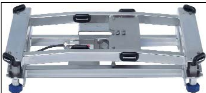
Typical model PBA430 sub-frame (tubular steel frame) / Sous-châssis typique du modèle PBA430 (châssis en acier tubulaire)
