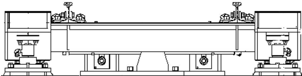
Cross sectional view of typical Model PL-XX-YY configuration / Vue en coupe, configuration typique du modèle PL-XX-YY
