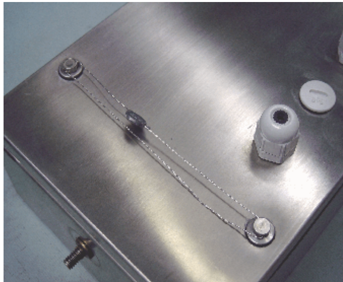
Typical Sealing Method / Méthode typique de scellage
