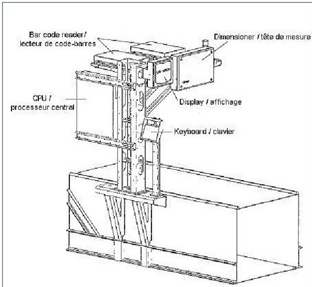
Typical Model CS900, CSN910 or CND910 / Modèle CS900, CSN910 ou CND910 typique
