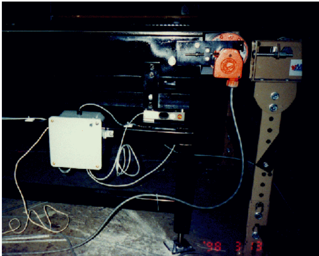
Junction box and load cell / Boite de jonction et cellule de pesage
