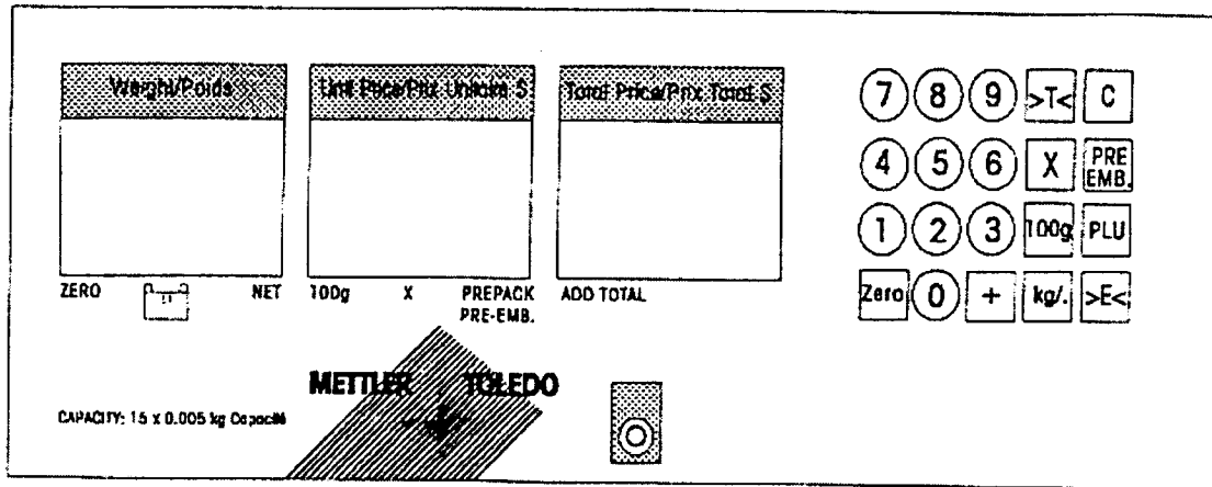
Operator display and keypad / Affichage de l'opérateur et clavier
