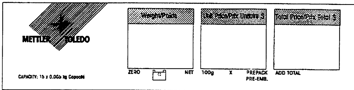
Customer display / Affichage du consommateur
