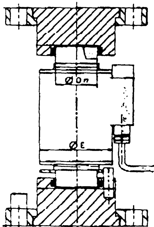
LOAD CELL MOUNTING/ Montage de la cellule de pesage
