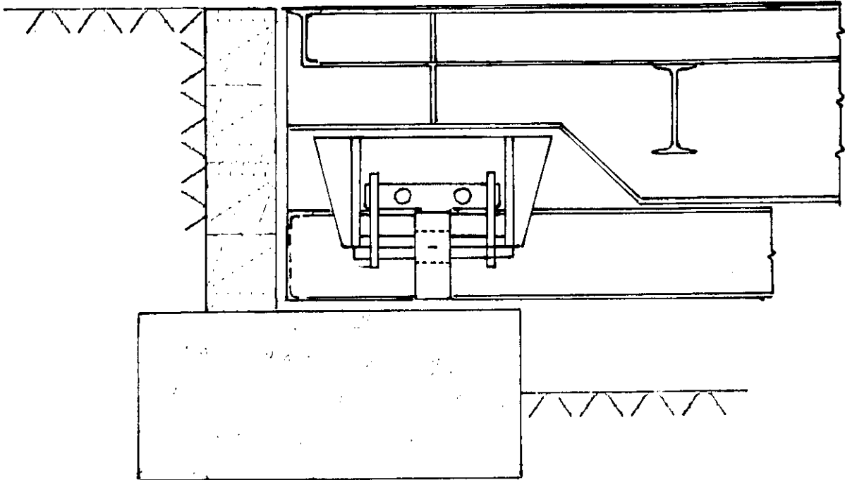
Load Cell Mount / Montage de la cellule de pesage
