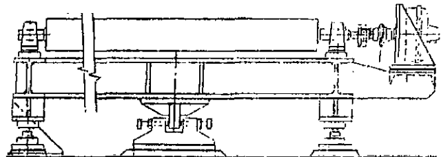
LOAD CELL AND SCALE RESTRAINT/ Cellule de pesage et contrainte de pont-bascule
