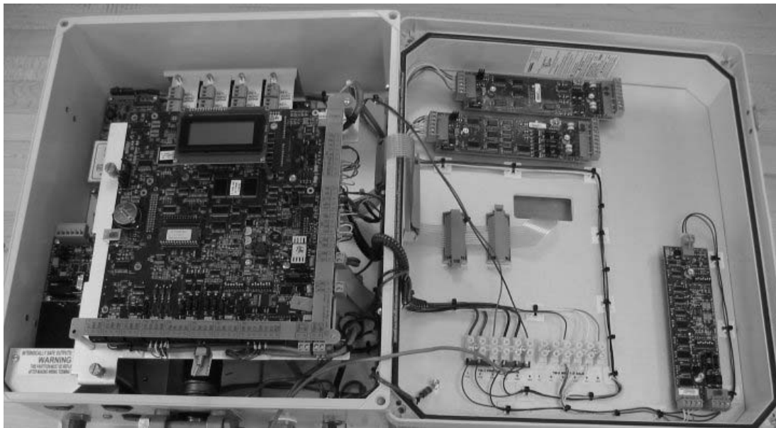
Fig. 9: AutoPilotPro with Analog Input Expansion and MEBs / AutoPilotPro avec extension d'entrées analogiques et CEM
