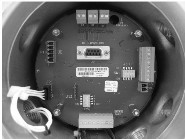
Fig. 3 : Termination Board / Carte de terminaison
