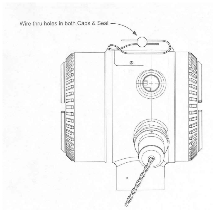
Fig. 6 : Sealing of Enclosure /Scellage du boîtier
