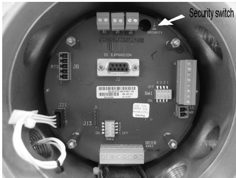
Fig. 7 : Location of Security Switch / Emplacement de l'interrupteur de sécurité
