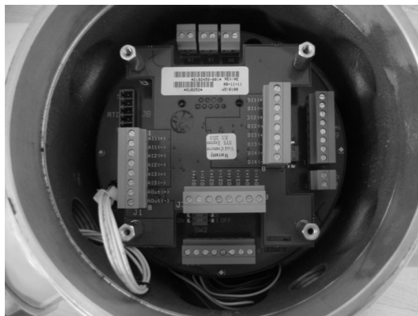
Fig. 4 : I/O Board / Carte E/S
