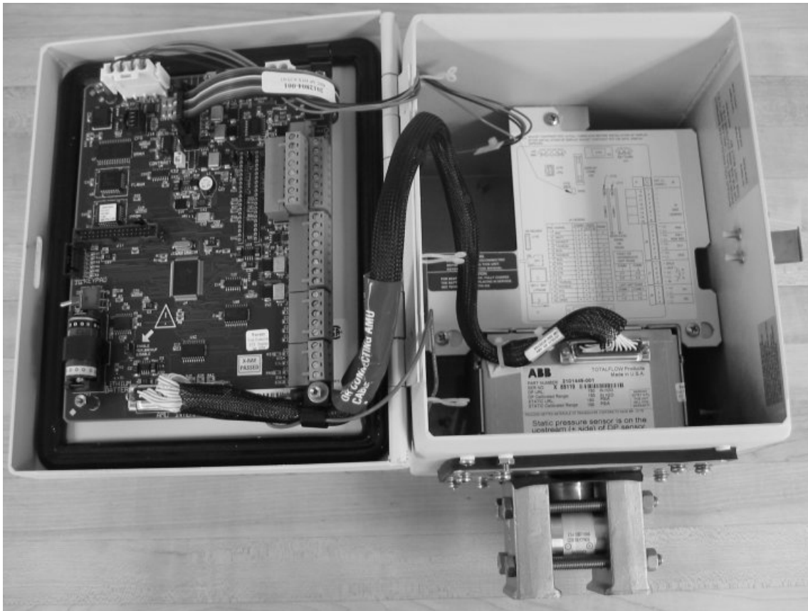
Fig. 2 : XFC 6410 (internal) / XFC 6410 (vue intérieure)
