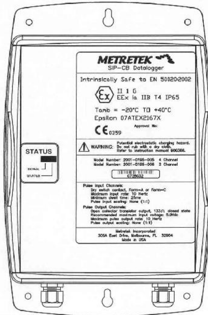
Fig. 1 : SIP-CB Data Logger, top cover / Couverture supérieure de l'enregistreur de données SIP-CB
