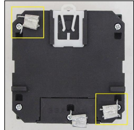
Figure 3 – 2 metrology seals on the underside of the display module. / 2 sceaux métrologiques sur le dessous du module d'affichage.
