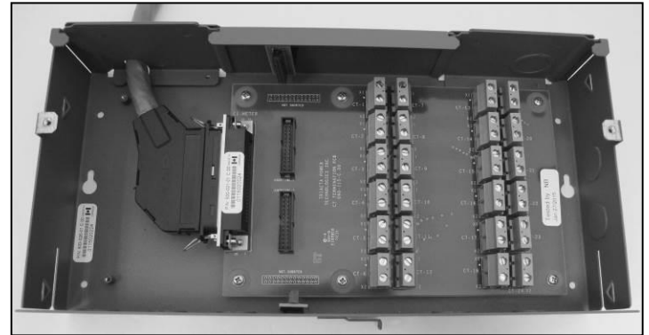
CT Termination Module / Module de connexion de transformateurs de courant
