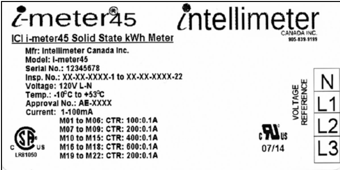
i-meter45 meter nameplate / Plaque signalétique du compteur i-meter45
