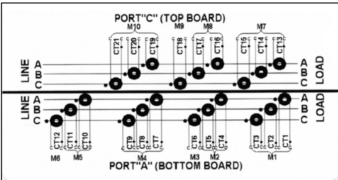
CT Box (ports) nameplate / Plaque signalétique de la « CT Box » (ports)
