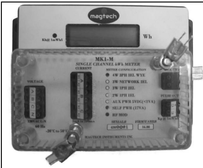
MK1-M meter with transparent terminal cover/ Compteur MK1-M avec couvre-bornes transparent
