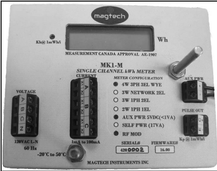
MK1-M nameplate / Plaque signalétique pour le MK1-M
