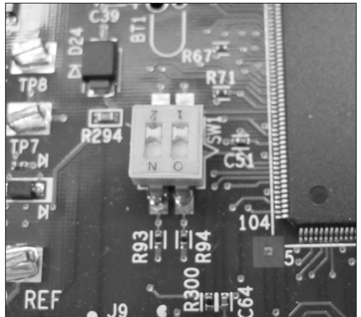
Programming Switch in Sealed Position 1-2 / Interrupteur de programmation en position scellée 1-2
