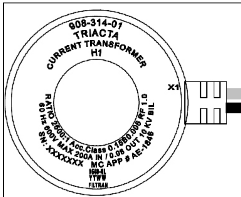
X1 - White Wire / X1 - Fil blanc
