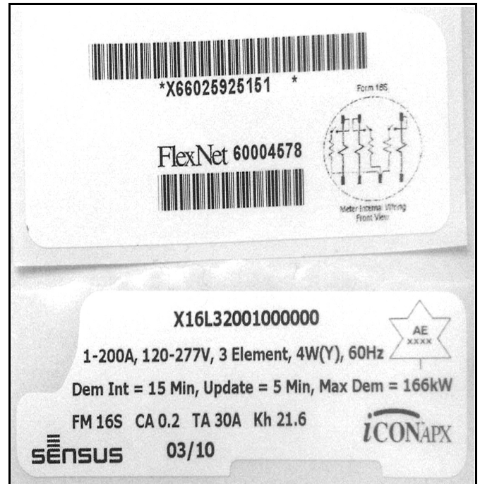
iCONAPX Nameplate with FlexNet / Plaque Signalétique de iCONAPX avec FlexNet
