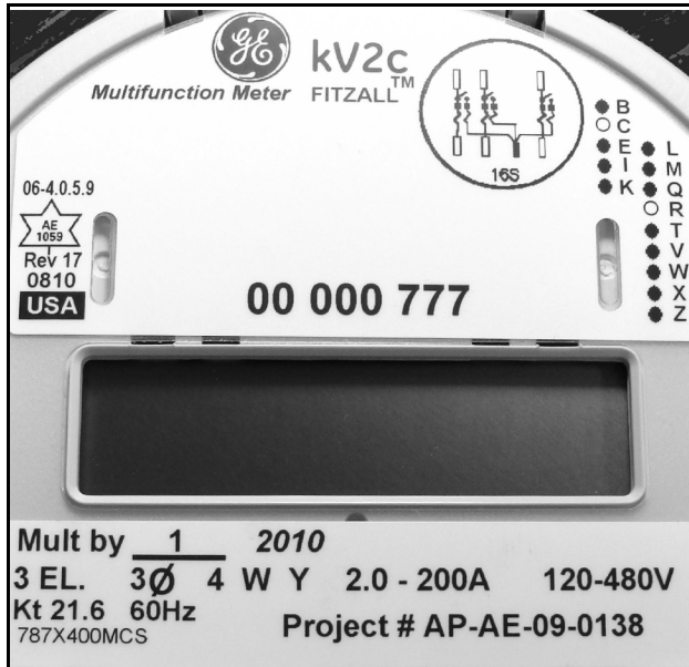
Nameplate for kv2c/ Plaque signalétique pour kv2c
