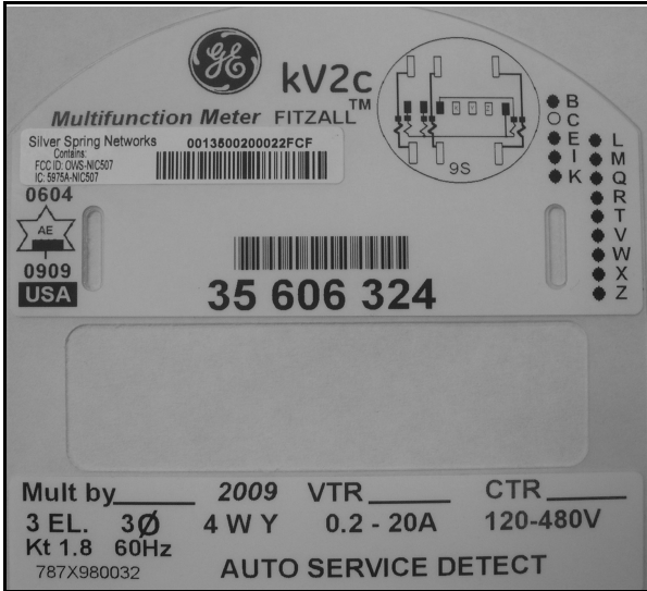
kv2c markings with new SSN module / Marquages de kv2c avec le nouveau module SSN
