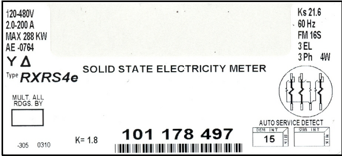
RXRS4e Demand Nameplate / Plaque Signalétique de puissance de RXRS4e
