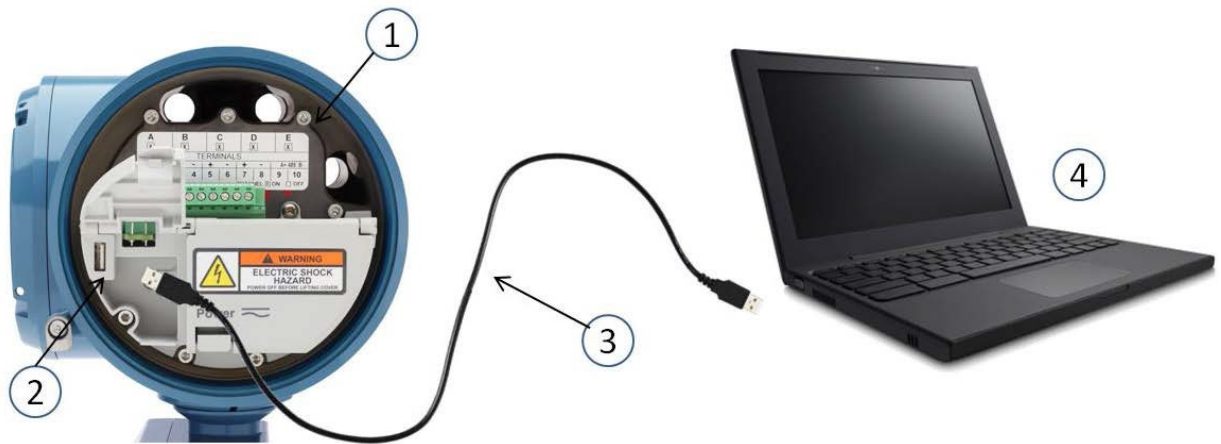
Figure 10: Accessing 5700 Transmitter parameters using ProLink: | Accès aux paramètres de transmetteur 5700 en utilisant le logiciel ProLink :
