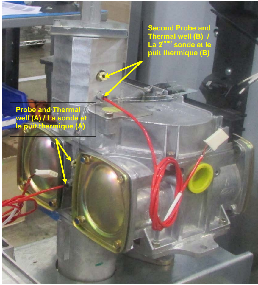
Figure 8: Location of the two ATC temperature probes and the corresponding thermal wells / Localisation des deux sondes de température du CAT et les puits thermiques correspondants.
