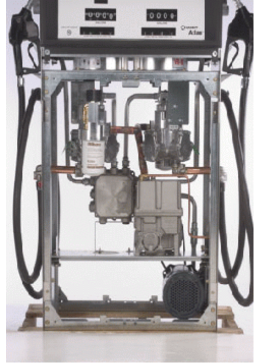
Atlas series dispenser model 87**K / Distributeurs de la série Atlas, modèle 87**K
