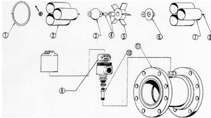
PT Series 1, 1.5, 2 and 2.5 inch turbine meter / Compteur turbine série PT 1, 1.5, 2, et 2.5 pouces
