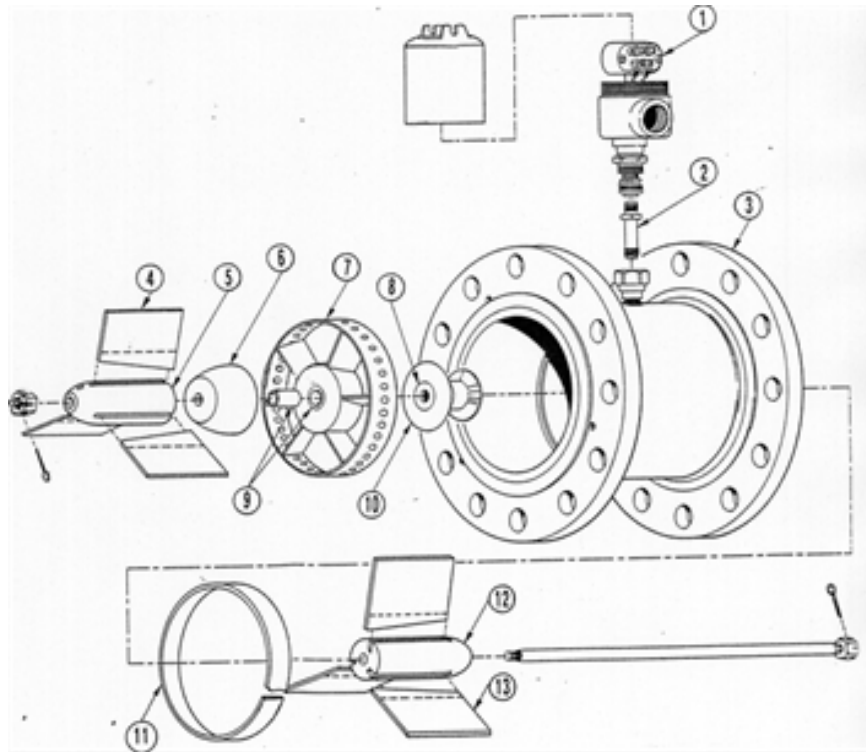
PT Series 3 and 4 inch turbine meter Compteur turbine série PT 3 et 4 pouces
