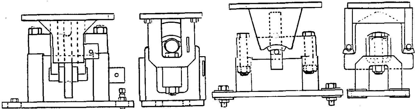
SADDLE LINK LOAD CELL MOUNT/Montage par anneau en selle
