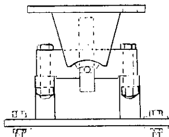
SADDLE LOAD CELL MOUNT/Montage par anneau en selle
