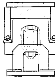
SADDLE LOAD CELL MOUNT/Montage par anneau en selle
