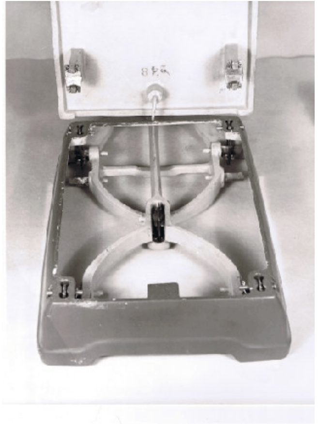
Typical lever system for both models SP900 and SP901/ Système de levier typique pour les modèles SP900 et SP901
