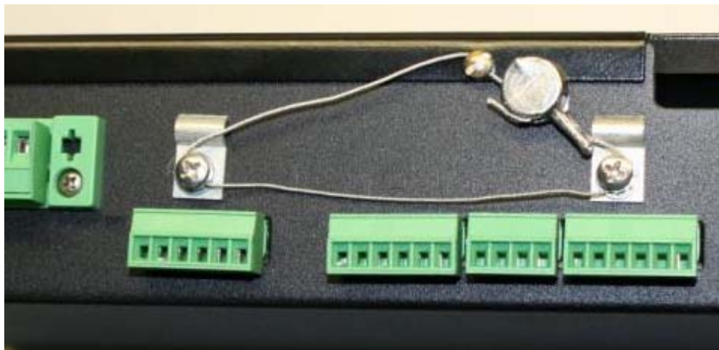
Sealing for models 720i-1A, 720i-1D and 720i-1E / Scéllage pour les modèles 720i-1A, 720i-1D et 720i-1E
