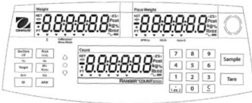
Typical RC31P*** display and keys / Affichage et touches typique du modèle RC31P***
