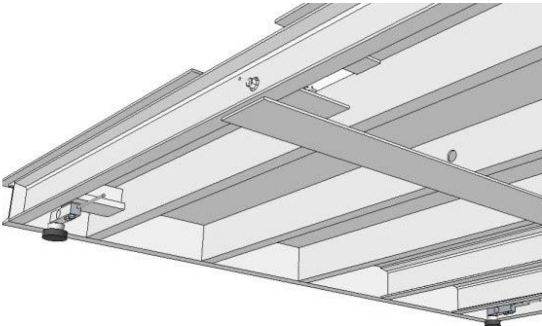
Subplatter and load cell mounting / Sous-plateau et le montage de la cellule de pesage
