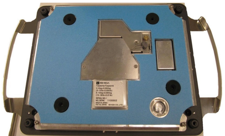
Typical sub-frame and sealing / Sous-chassis et scellé typique.
