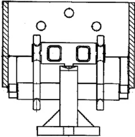
Load cell mounting system / Montage des cellules de pesage
