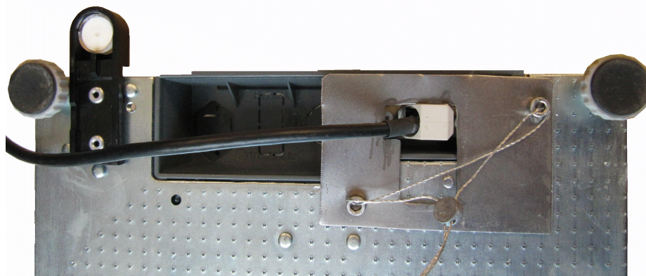
Typical sealing of load cell cable of model K 100 G / Scellage typique du câble de la cellule de pesage du modèle K 100 G
