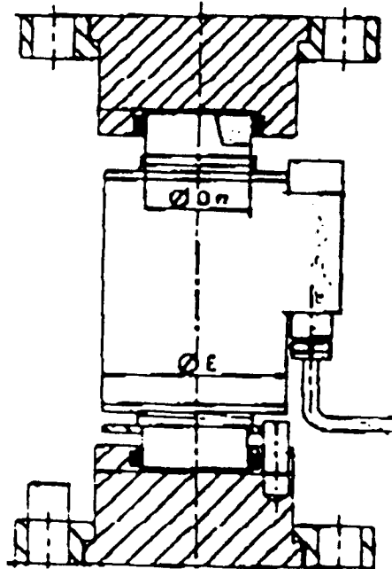
LOAD CELL MOUNTING/ Montage de la cellule de pesage
