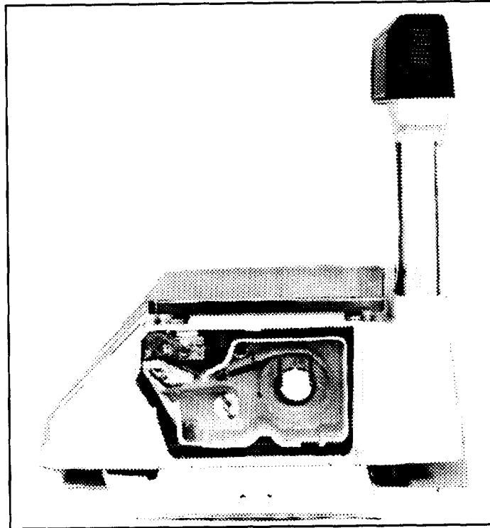
SIDE VIEW / vue de côté
